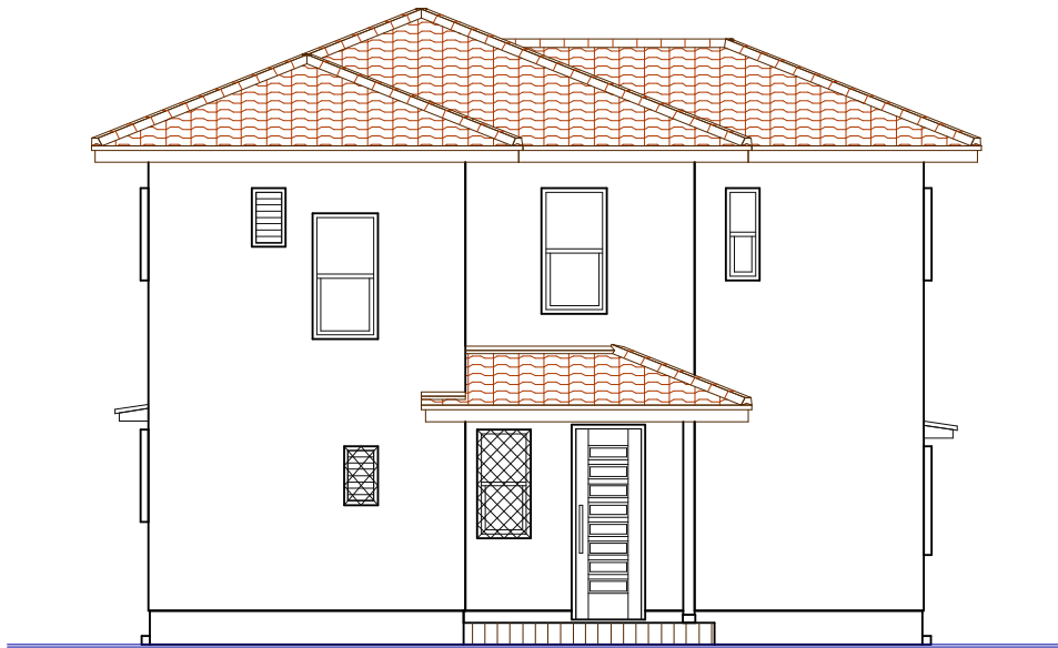
北側立面図
