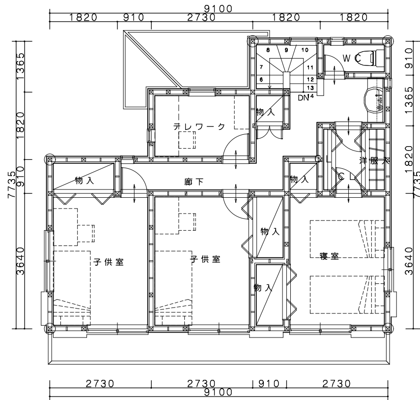
2階平面図
