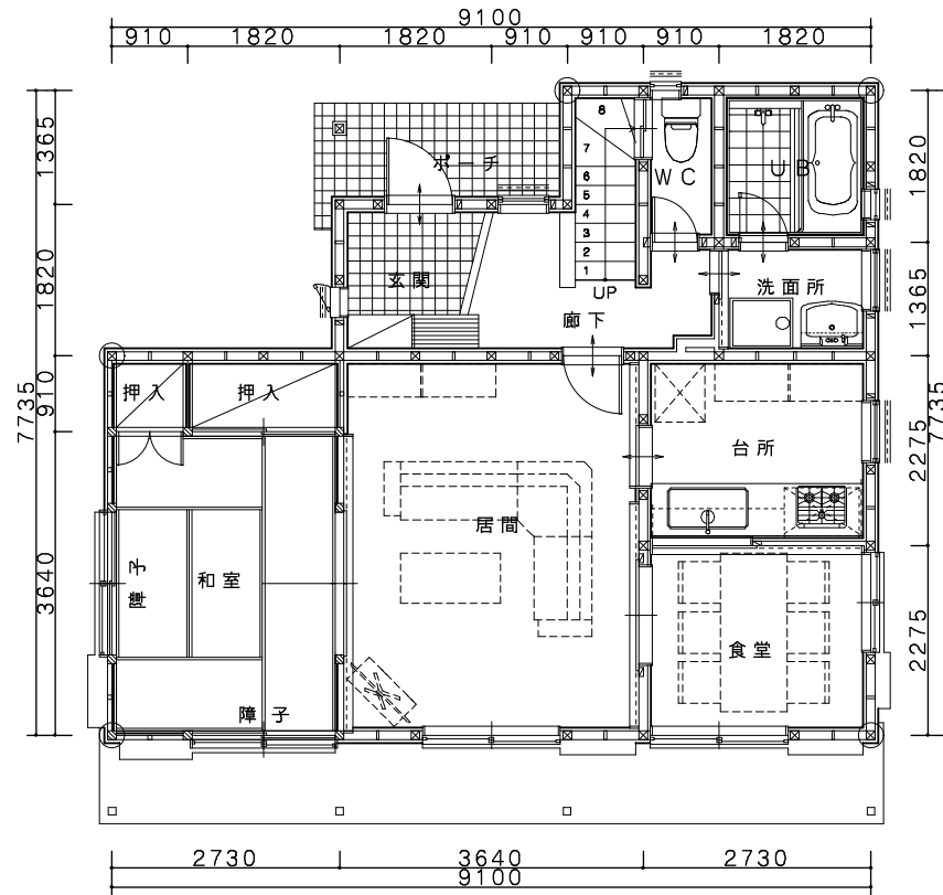
1階平面図
