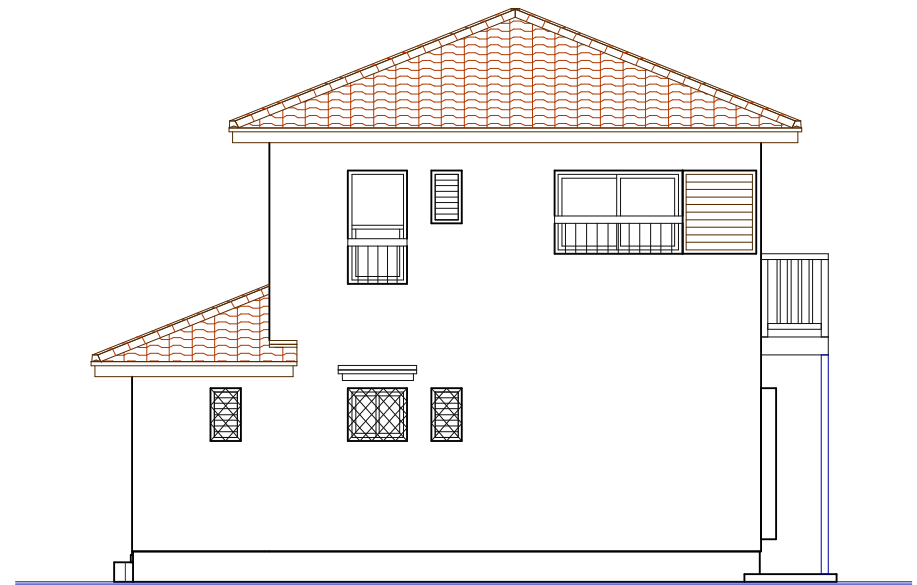
西側立面図
