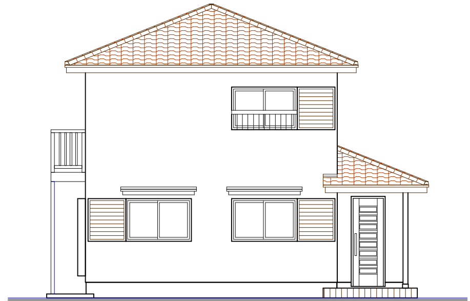
東側立面図
