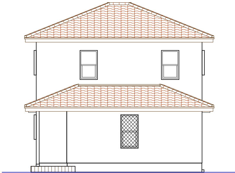
北側立面図
