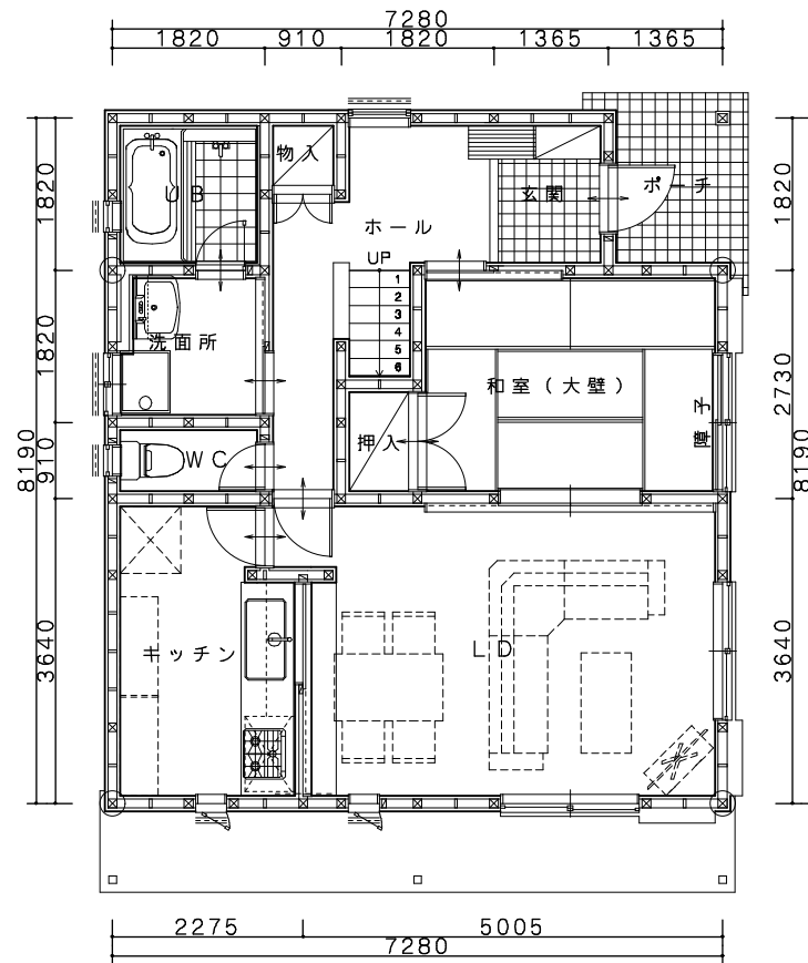
1階平面図
